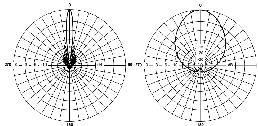
Диаграммы направленности антенны RFE 2700/60/18MIMO.
